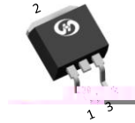
TO-263
